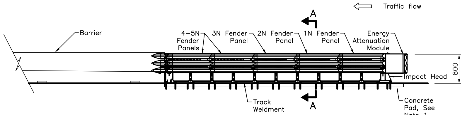
ELEVATION
